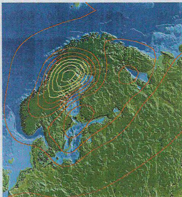
3c. 100 ka. OIS-5c. Brorup interstadial
