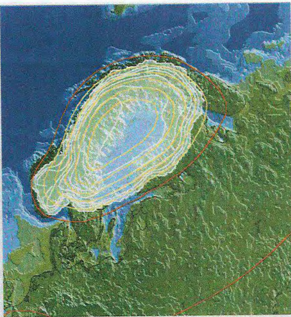
4b. 57 ka. OIS-3. Moerhoofd interstadial (Maximum ice limits)
