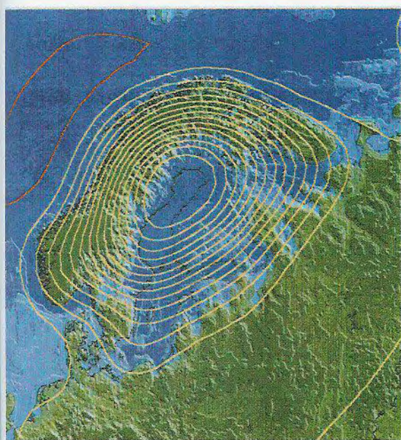
3a. 129 ka. OIS-5e. Early Eemian
